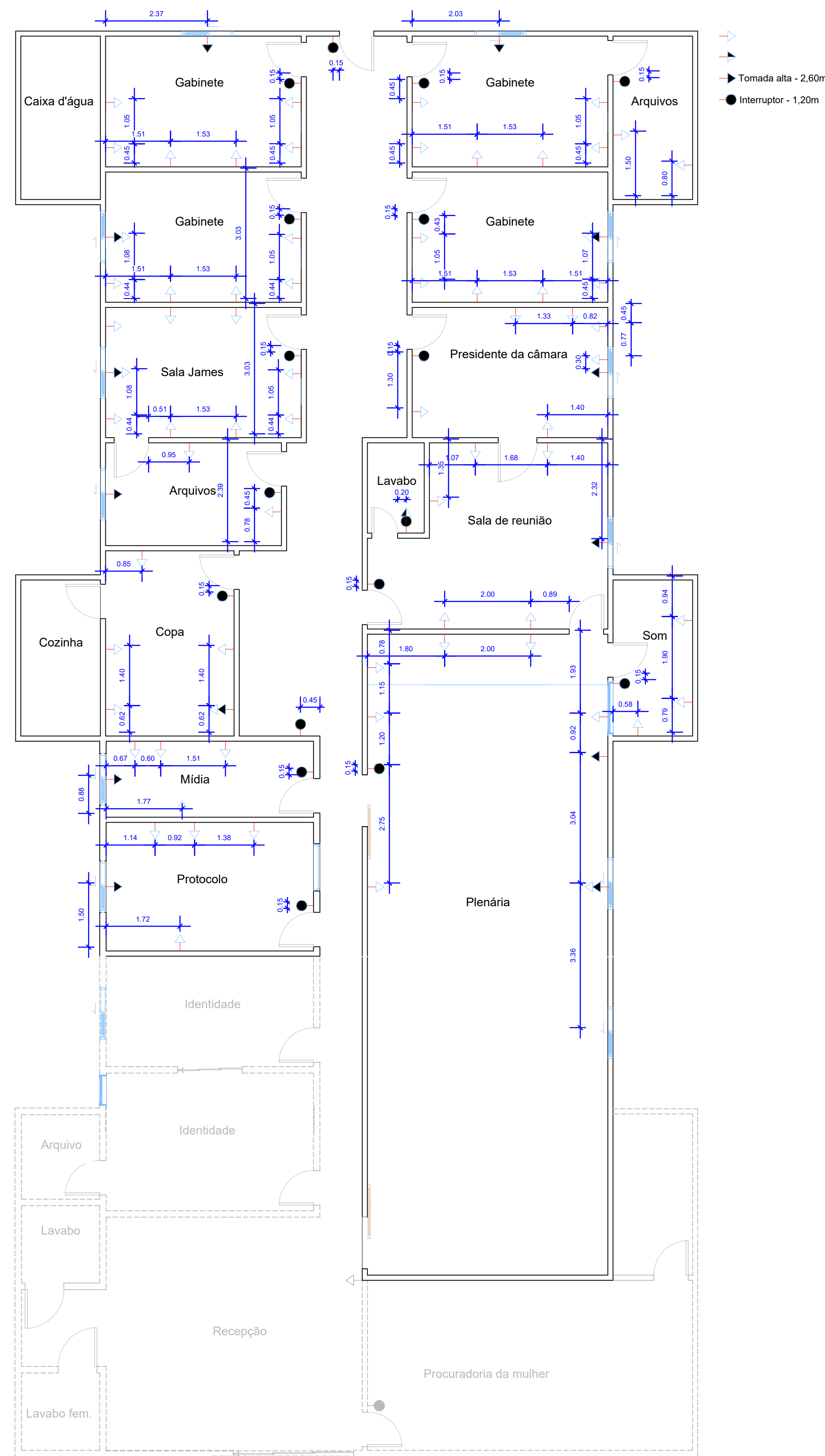
03 PONTOS ELÉTRICOS ESC: 1/75
